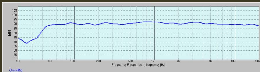
スピーカーシステム周波数特性 (35Hz 以下の応答は暗騒音によるものです)
